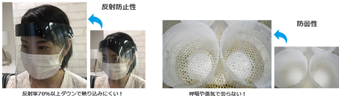
■200回拭き取り試験後の各種特性
